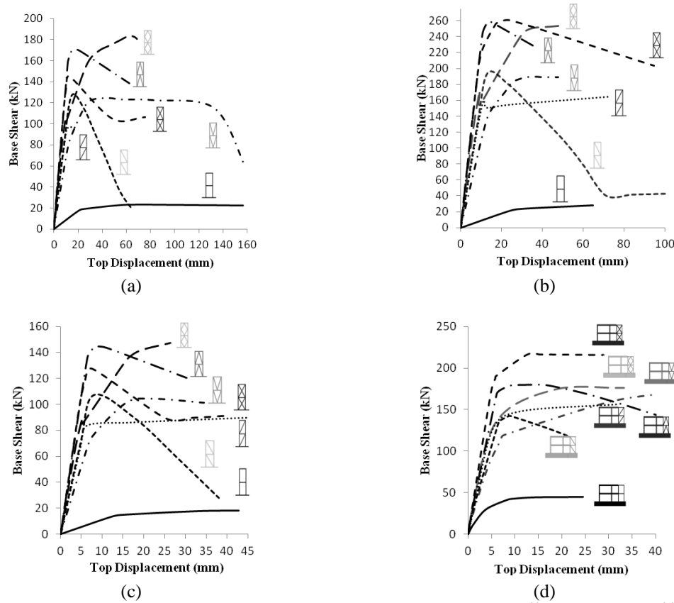
Fig. 8 Lateral load-carrying capacities of CSBF types: (a) 1/2\text{CSBF}^{(-)} ; (b) 1/2\text{CSBF}^{(+)} ; (c) 1/3\text{CSBF}^{(+)} ; (d) 1/3\text{RC}+\text{CSBF}^{(+)}
